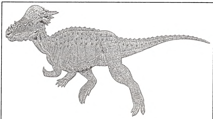
Пахицефалозавр
